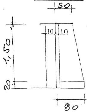
SEZ. 4
