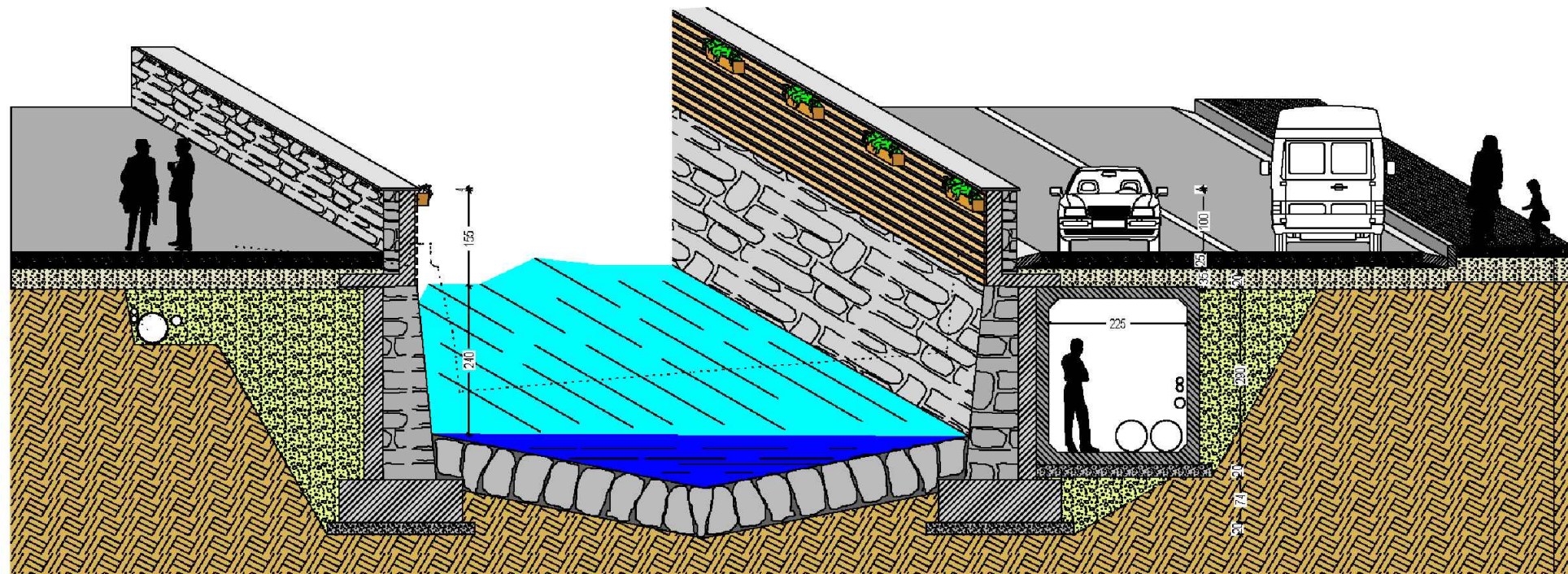
SEZIONE TIPO SCALA 1/100
